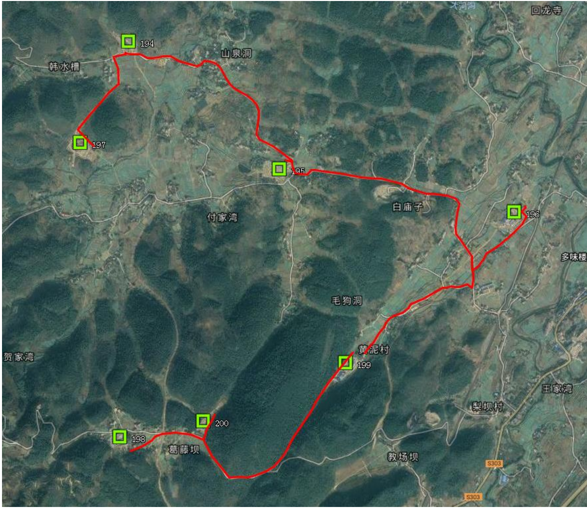
图 6.1-1 工区废水收集及利用临时管网走向图
