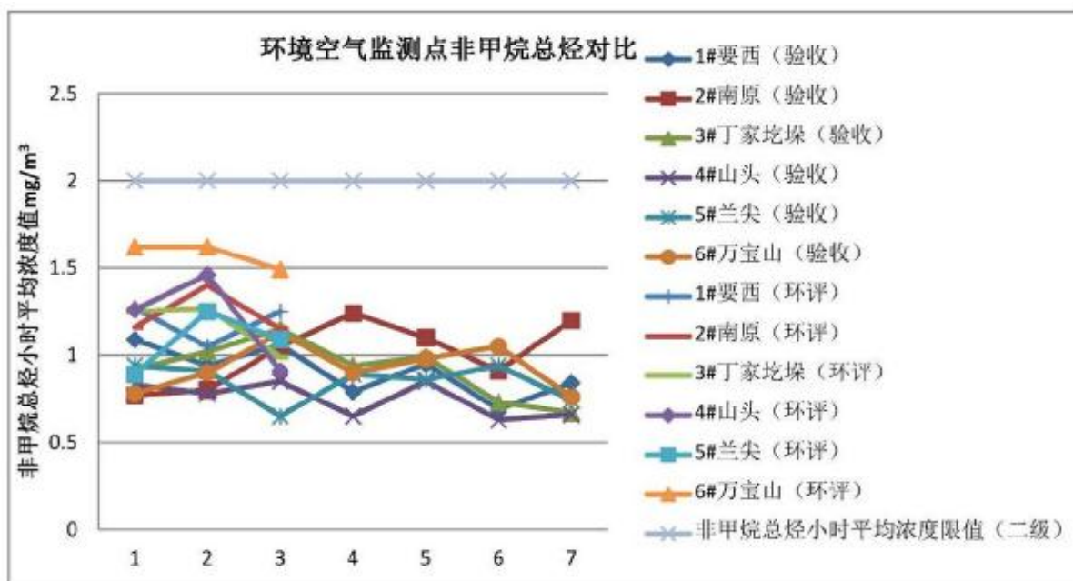
图 8-3-5 环境空气监测点非甲烷总烃 2:00 对比图 (验收、环评、浓度限值)
