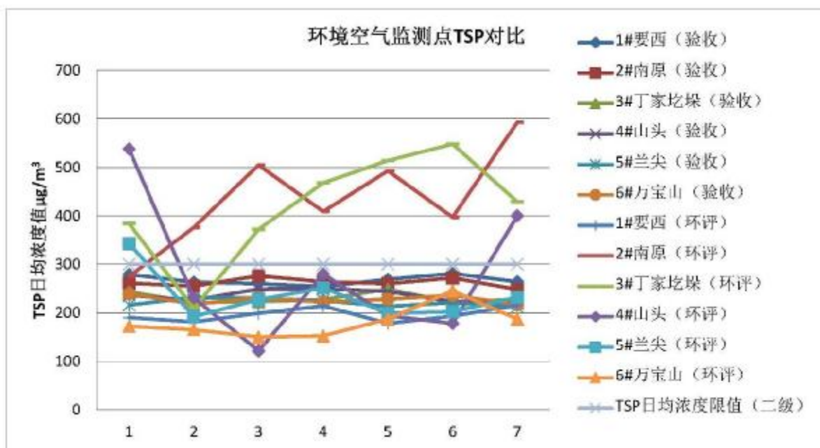
图 8-3-1 环境空气监测点 TSP 对比图 (验收、环评、浓度限值)
