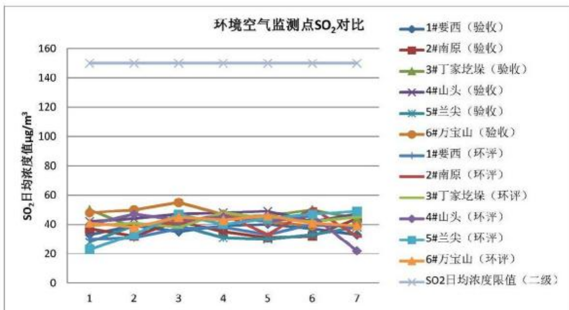
图 8-3-4 环境空气监测点 SO 2 对比图 (验收、环评、浓度限值)
