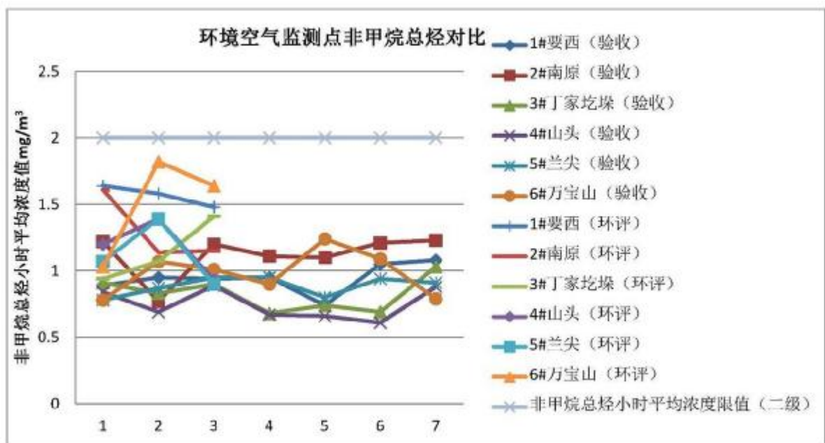
图 8-3-6 环境空气监测点非甲烷总烃 8:00 对比图 (验收、环评、浓度限值)
