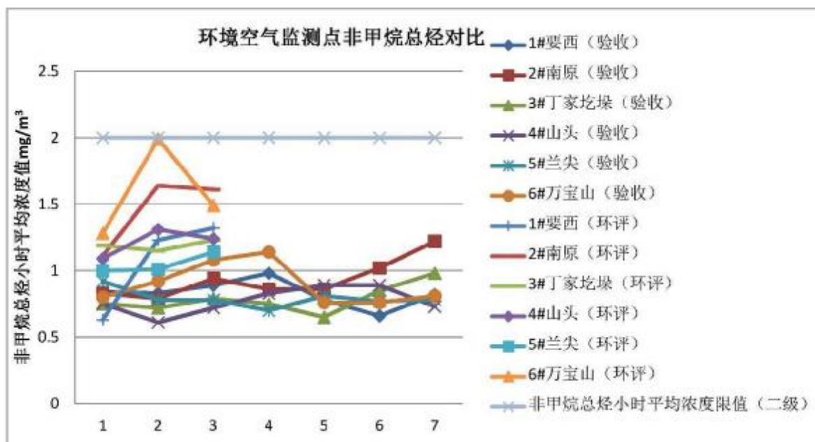
图 8-37 环境空气监测点非甲烷总烃 14:00 对比图（验收、环评、浓度限值）
