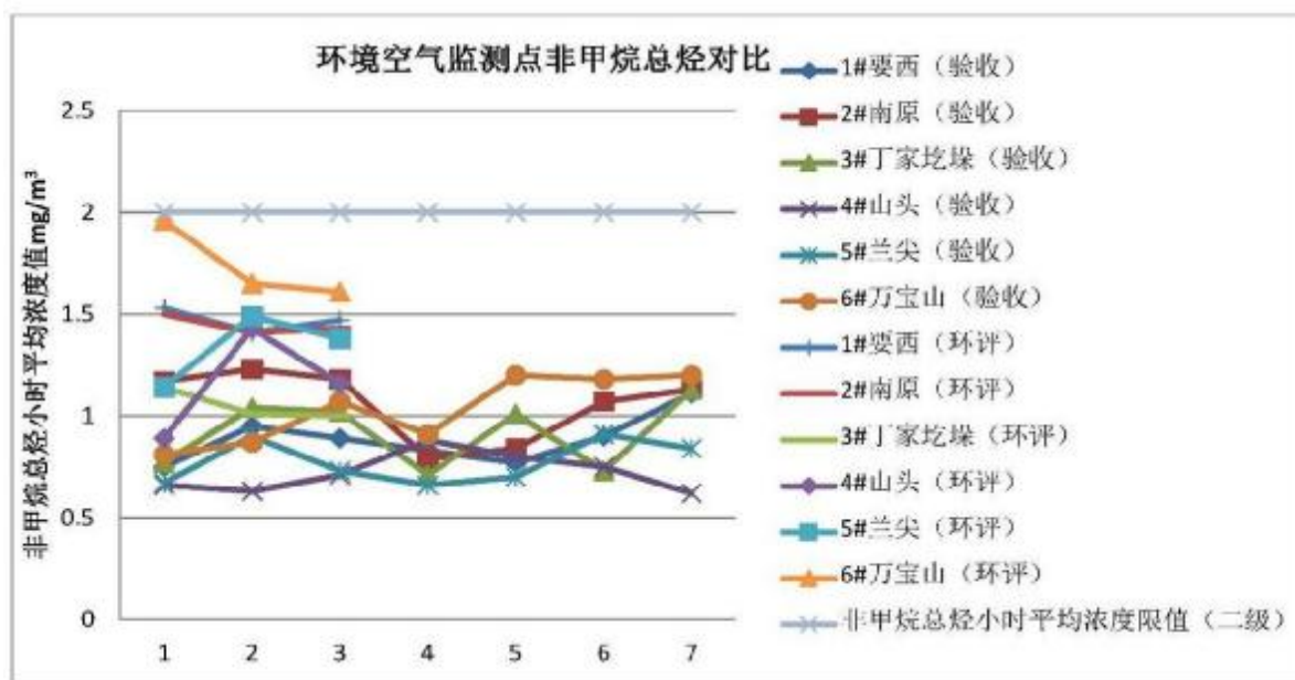
图 8-3-8 环境空气监测点非甲烷总烃 20:00 对比图（验收、环评、浓度限值）
