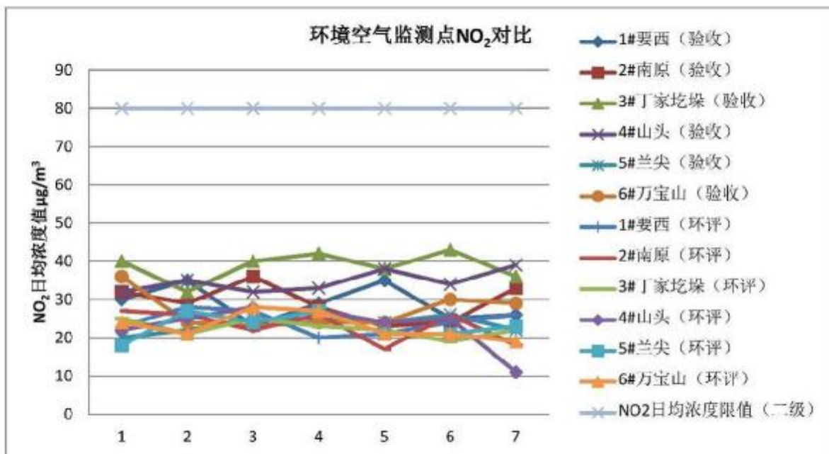
图 8-3-3 环境空气监测点 NO 2 对比图 (验收、环评、浓度限值)
