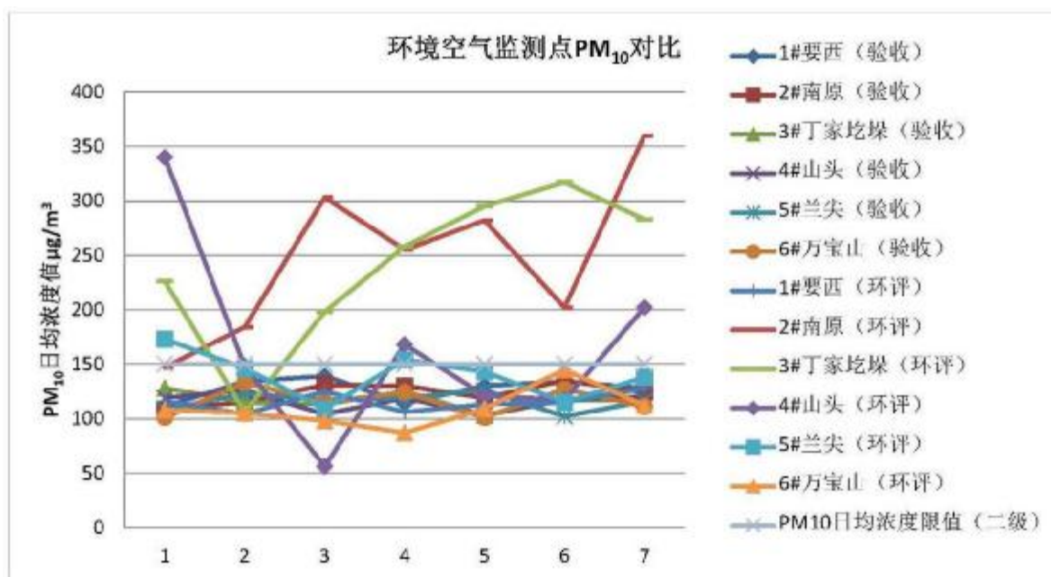
图 8-3-2 环境空气监测点坡面 PM 10 对比图 (验收、环评、浓度限值)
